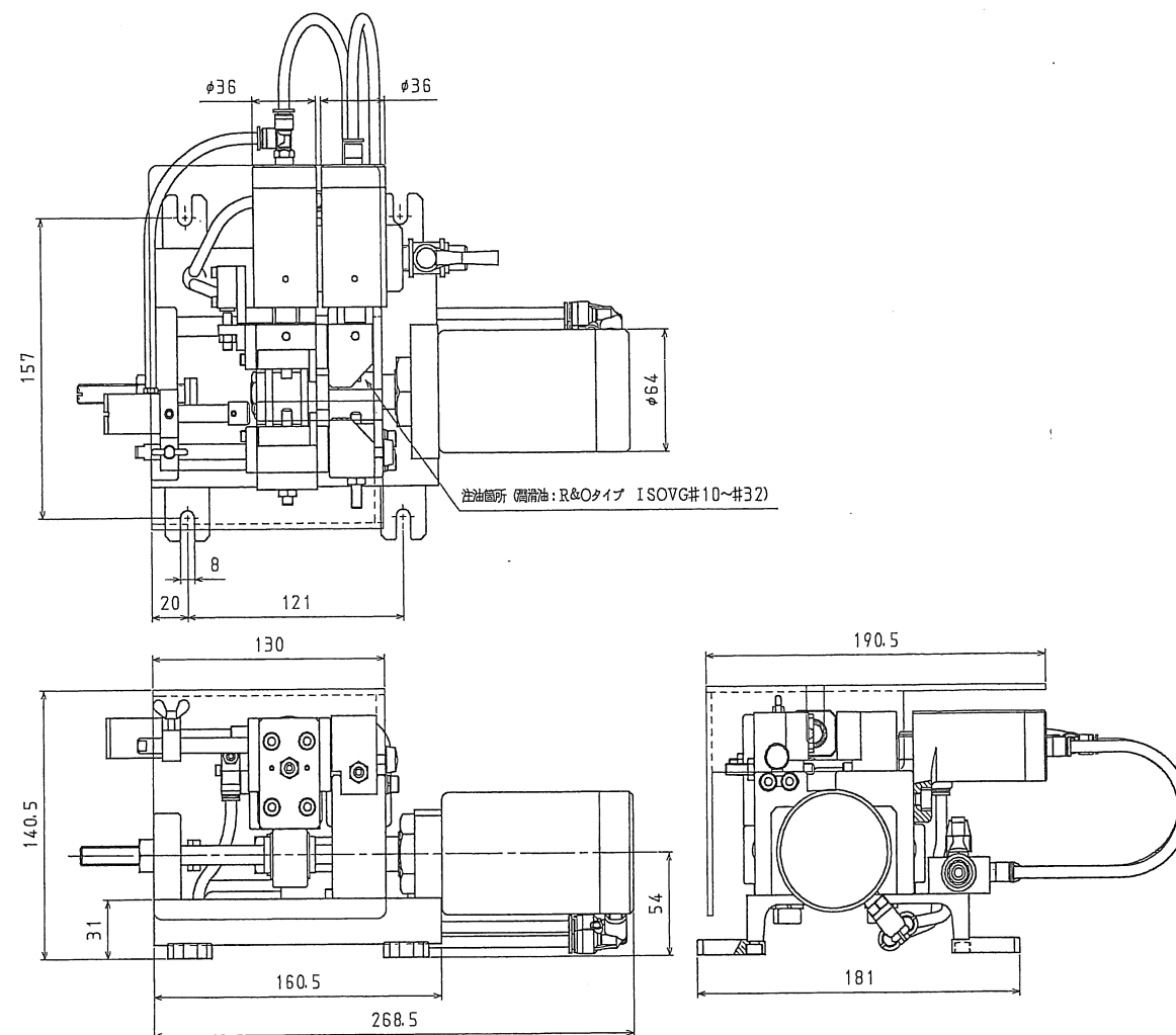
外観寸法図
