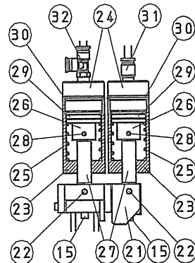
ツカミ部、替刃部シリンダー断面図
