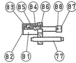
アタリシリンダー断面図
