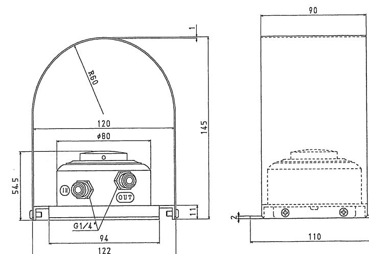
付属品 フットバルブ：FB70S 外観寸法図
