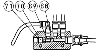
チェック弁断面図
