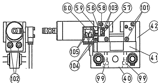
替刃部
