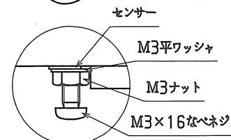
センサー取付部詳細図 (取付部品は替刃付属品)
