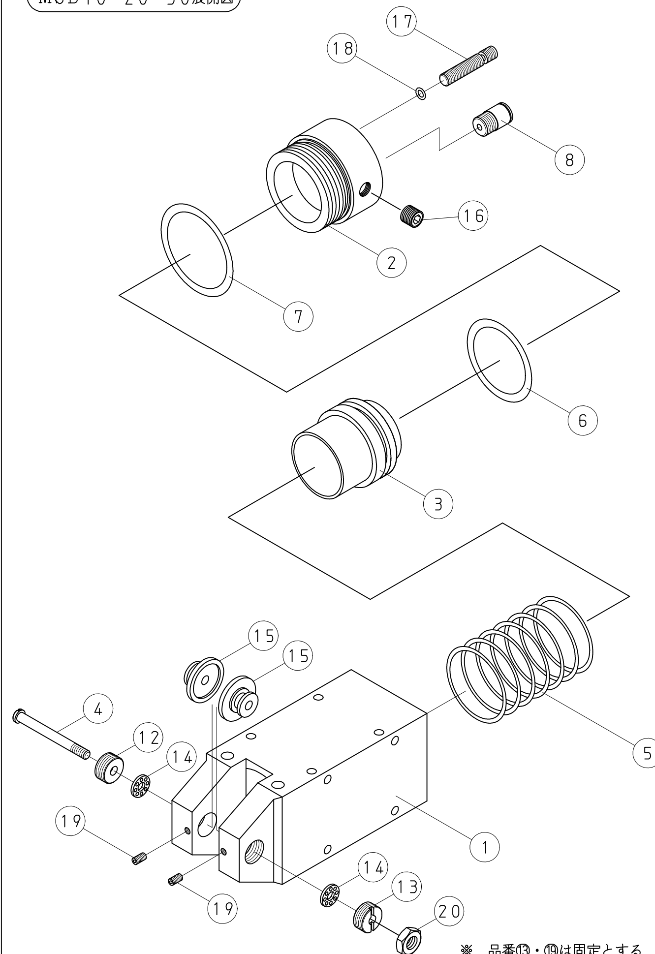
MSB10・20・30展開図
