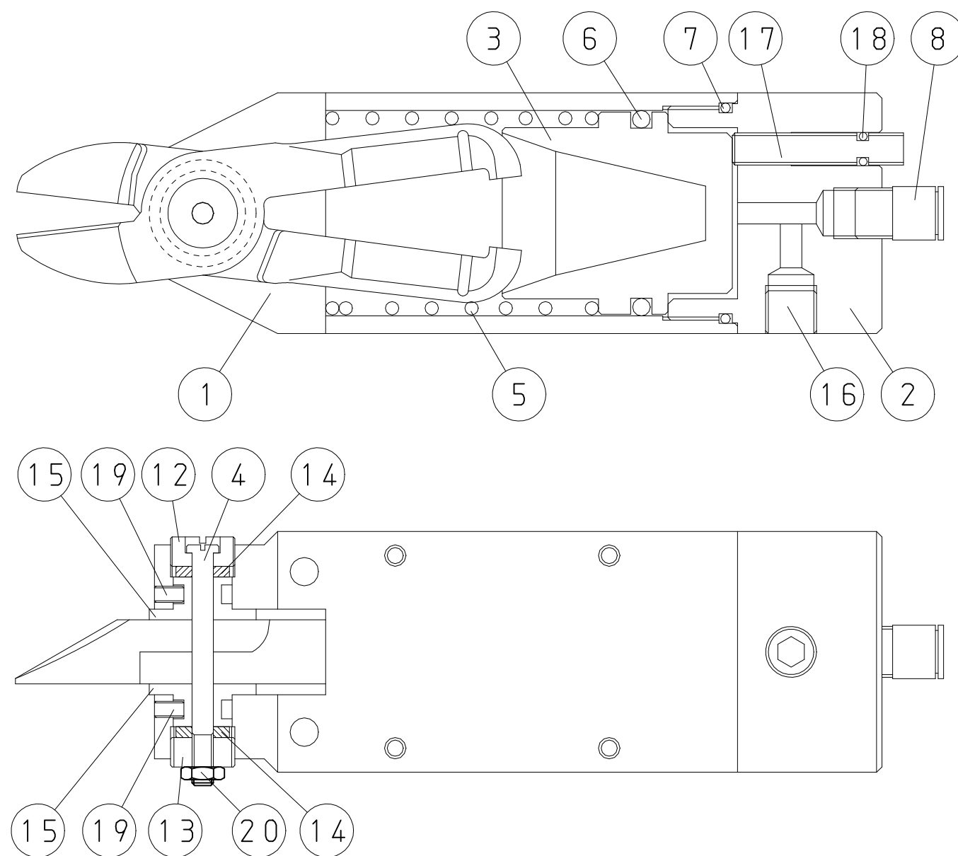
MSB10・20・30組立図
